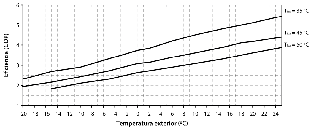
Curvas de eficiencia en calentamiento Dual Clima 16T (COP)
