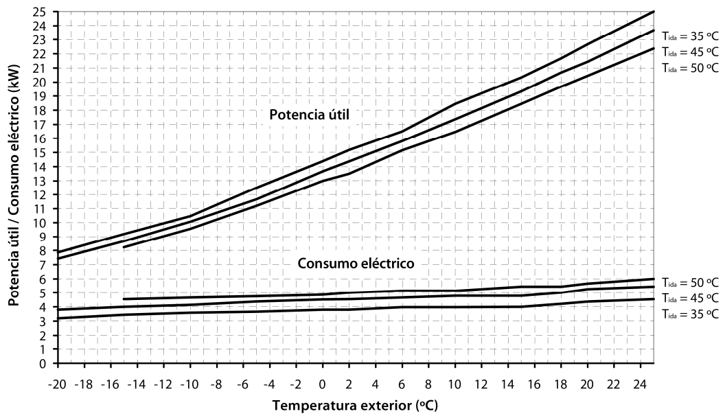
Curvas de prestaciones en calentamiento Dual Clima 16T
