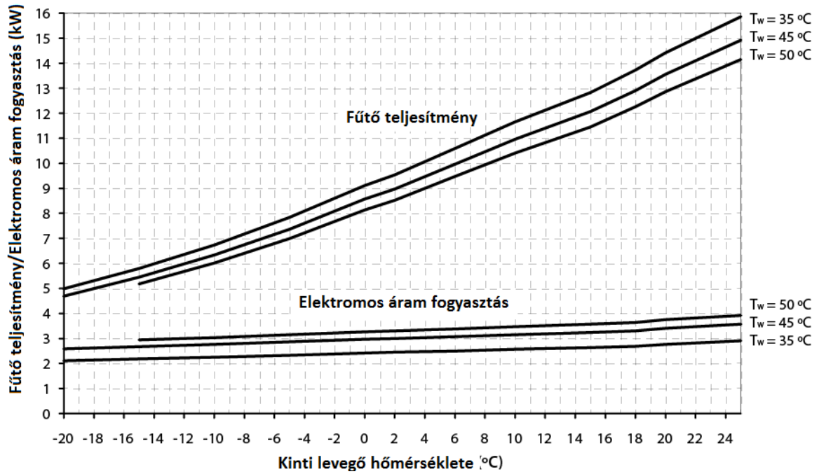
Dual Clima 11 fűtési teljesítmény görbéje
