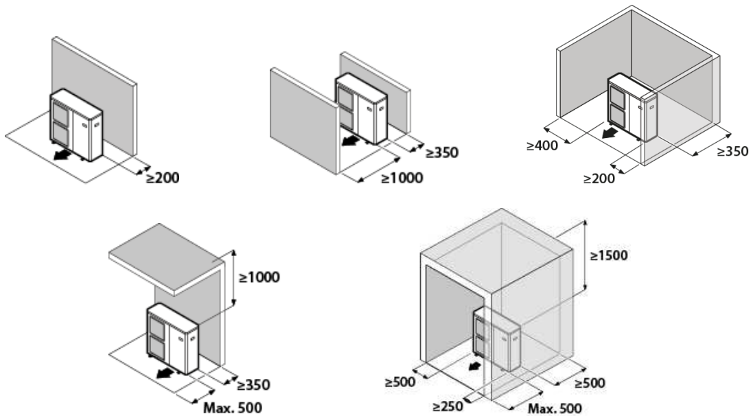
Minimumafstanden voor de installatie van één eenheid (mm).
