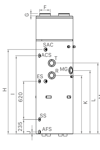
ACHTERAANZICHT HYDREA 280
