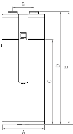
VOORAANZICHT HYDREA 150
