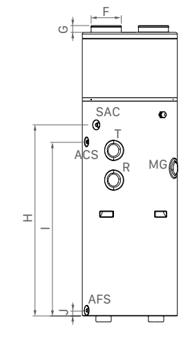
ACHTERAANZICHT HYDREA 200
