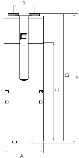
VOORAANZICHT HYDREA 200 / HYDREA 280
