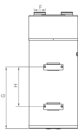
ACHTERAANZICHT HYDREA 150
